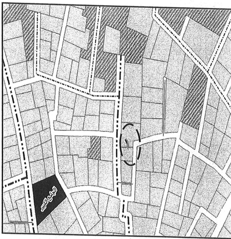
المخطط التفصيلي لقرية أبو داوود
