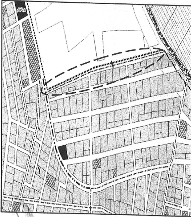
المخطط التفصيلي لقرية الخمسة
